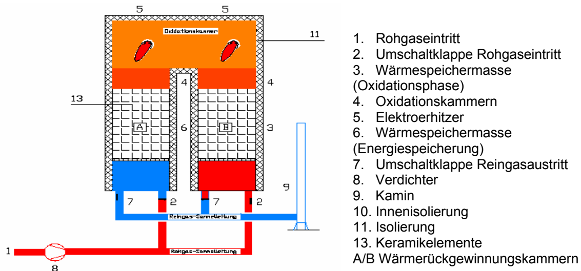
Abbildung. 15: Verfahrensschema der Nachverbrenung im DEPOTHERM®-Reaktor (Druckbetrieb) [UMAT 2005]
