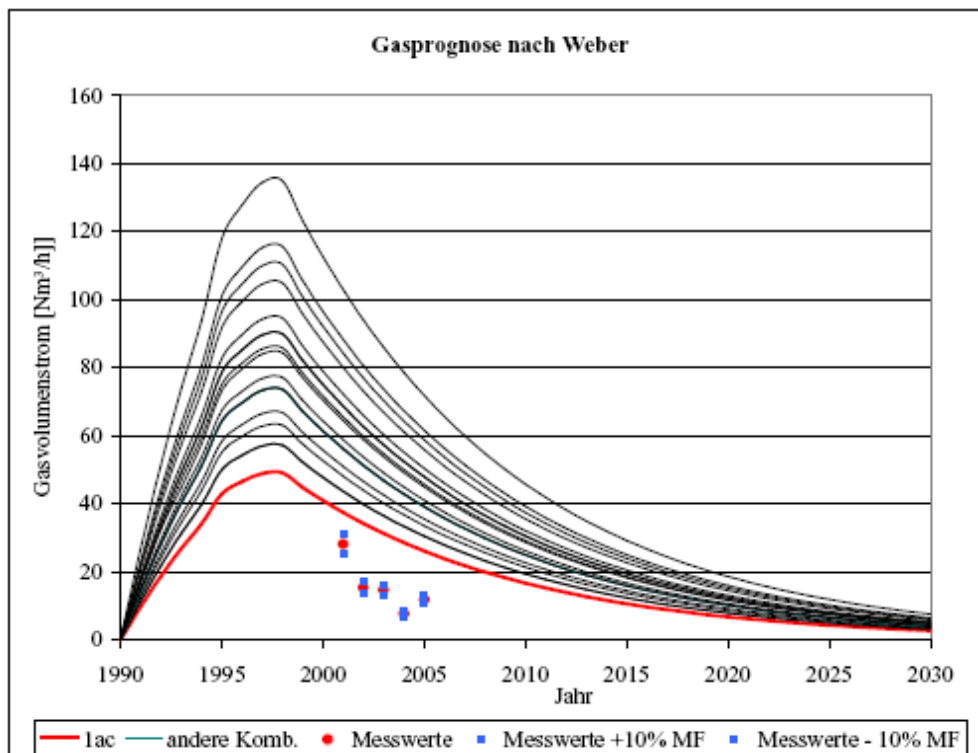
Abbildung 11: Gasprognosen nach Weber für die Deponie Penig
